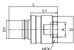
Innengewinde
