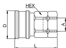
Innengewinde
