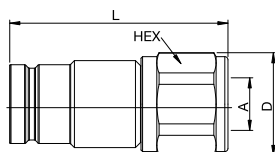
Innengewinde
