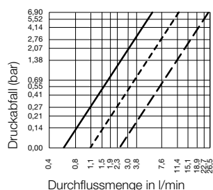
Druckabfall-Diagramm für Wasser
