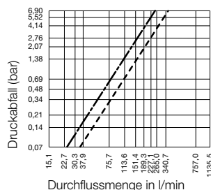
Druckabfall-Diagramm für Hydraulikmedium MIL-H-6083 bei 32°C +/-1,5°C
