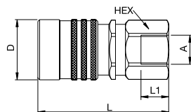
Innengewinde
