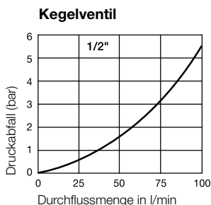
Druckabfall-Diagramm für Öl mit Viskosität 43cSt bei 38°C gemäß ISO 7241/2-2000
