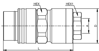
Innengewinde - BSPP
