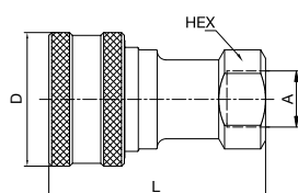
Innengewinde
