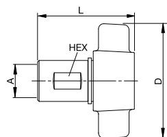
Innengewinde
