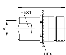
Innengewinde - mit Flansch
