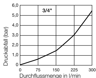
Druckabfall-Diagramm für Öl mit Viskosität 43cSt bei 38°C gemäß ISO 7241/2-2000
