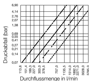
Druckabfall-Diagramm für Hydrauliköl 88 SSU mit Viskosität 18cSt
