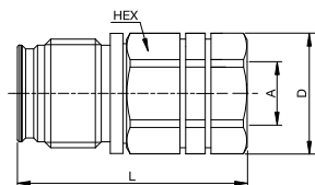
Innengewinde - BSPP
