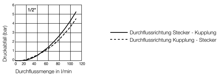
Druckabfall-Diagramm für Öl mit Viskosität 43cSt bei 38°C gemäß ISO 7241/2-2000
