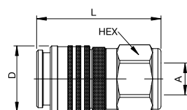
Innengewinde
