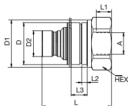
Innengewinde (ausgestattet mit Sicherungsring gemäß DIN 471)
