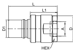
Innengewinde
