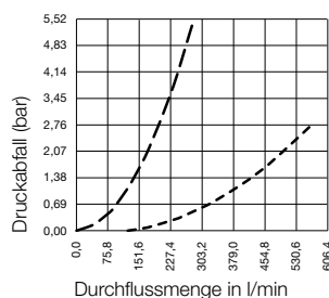
Druckabfall-Diagramm für Hydrauliköl mit Viskosität 30cSt
