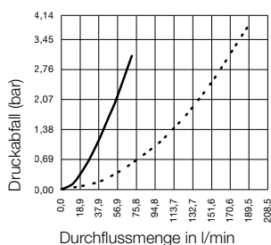
Druckabfall-Diagramm für Hydrauliköl mit Viskosität 30cSt
